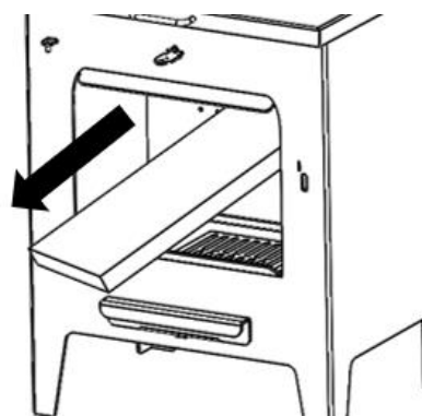
Figure n°16 - Extraire le déflecteur en le positionnant comme sur l'image
