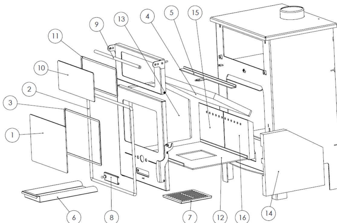
Figure n°19 - Pièces détachées Azur CH
