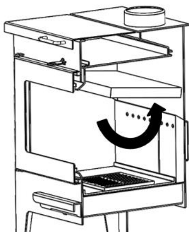
Figure n°11 - Faire pivoter le déflecteur vers le haut par l'arrière et le laisser relevé horizontalement
