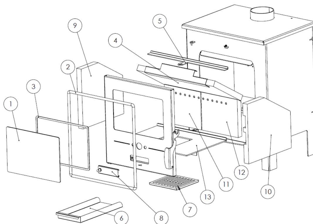
Figure n°17 - Pièces détachées Azur
