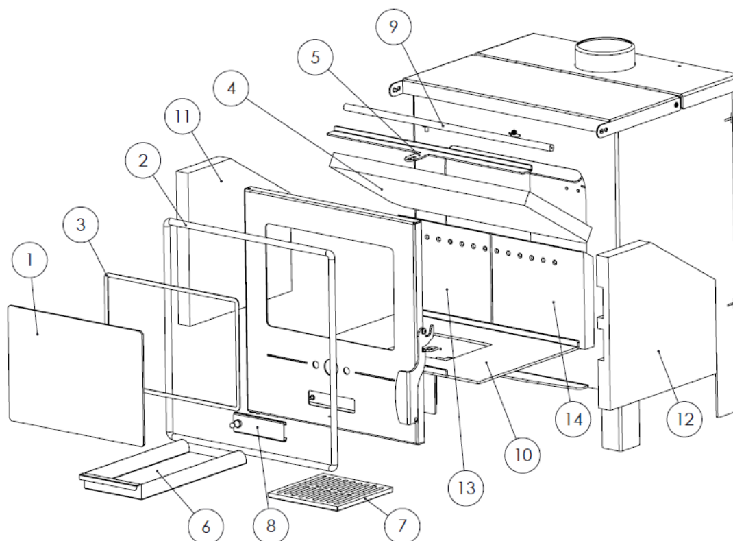
Figure n°18 - Pièces détachées Azur CP
