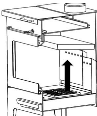
Figure n°12 - Soulever la vermiculite arrière gauche
