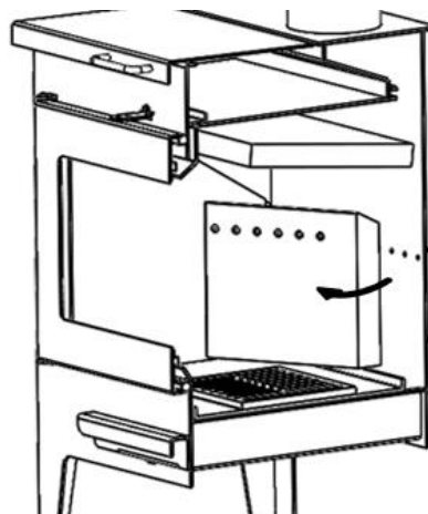
Figure n°14 - Extraire la vermiculite arrière droite
