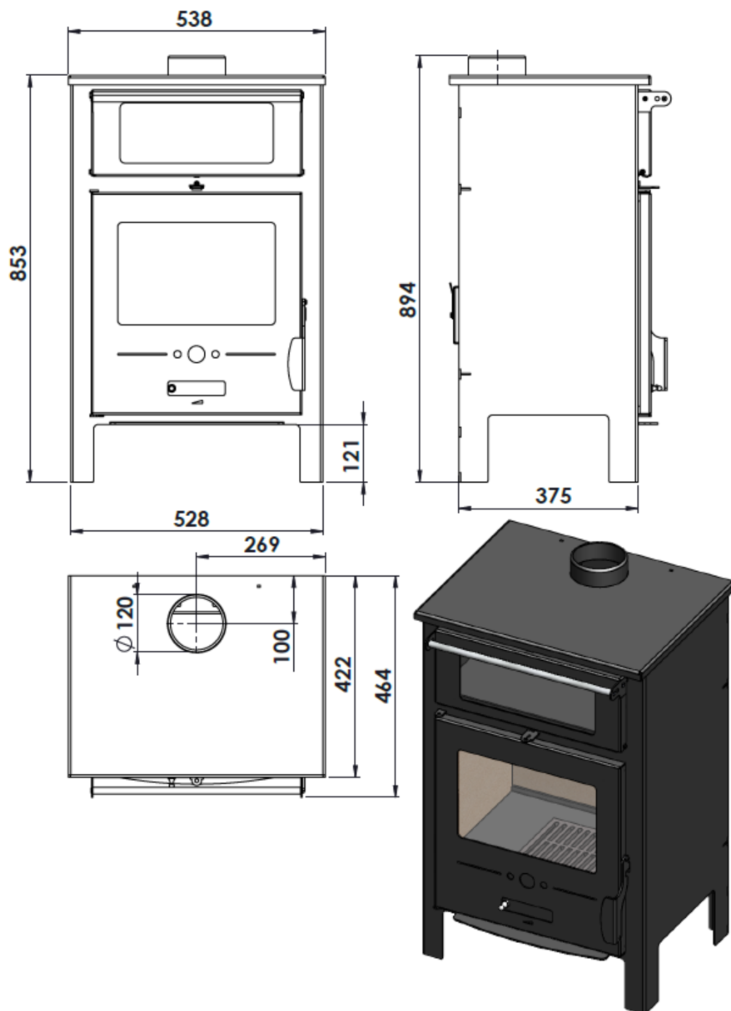
Figure n°3 - Dimensions en mm de l'appareil Azur CH
