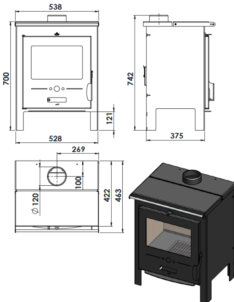
Figure n°2 - Dimensions en mm de l'appareil Azur CP
