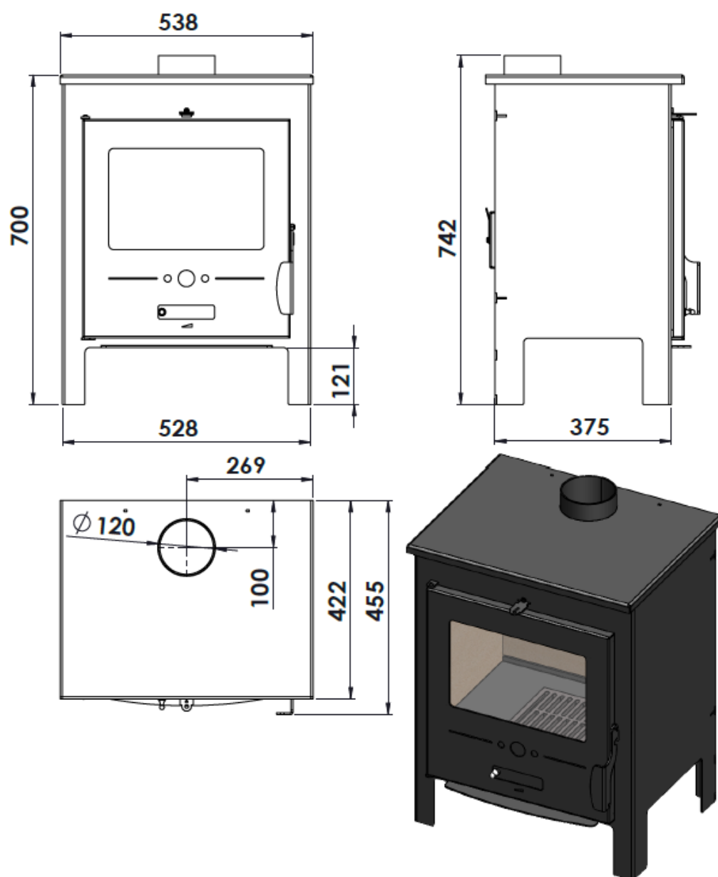
Figure n°1 - Dimensions en mm de l'appareil Azur
