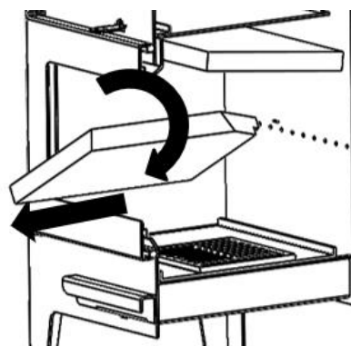
Figure n°15 - Tourner la vermiculite latérale gauche dans le foyer et l'extraire du foyer
